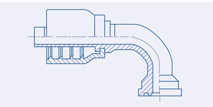
90° Elbow SuperCAT Flange - SC90
