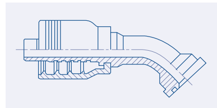
45° Elbow SuperCAT Flange - SC45
