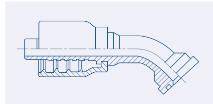
45° Elbow SuperCAT Flange - SC45
