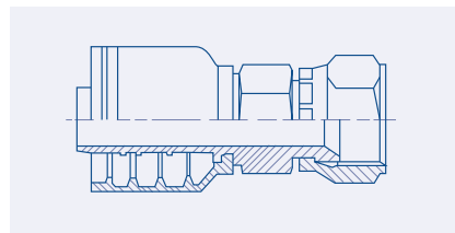
JIS 30° Female Swivel - JIS BF21.3712. pag. 55
