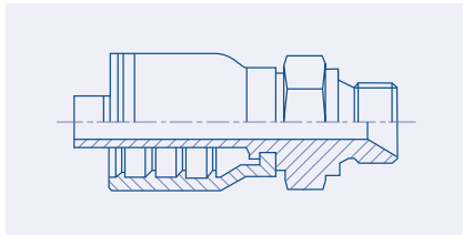
Light 24° Metric Male - DLM BF21.1000. pag. 48
