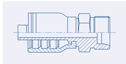
Heavy 24° Metric Male - DHM BF21.1100. pag. 52
