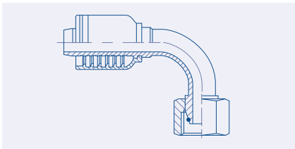
Light 24° Metric 90° Elbow Female - DLF90 BF21.5093. pag. 47
